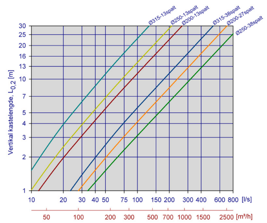
Diagram 11, kastelengde Tellus-LØV-S, -3gr.
