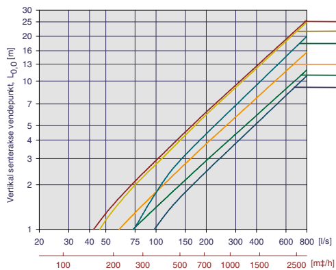
Diagram 14, kastelengde Tellus-LØV-S, +10gr.
