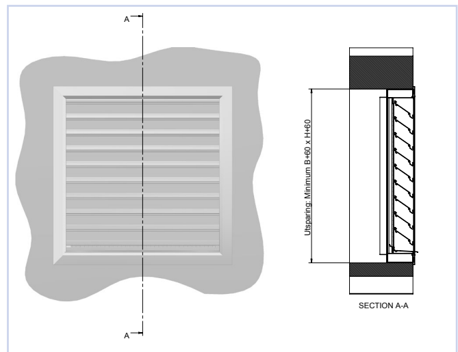
Figur 8, RIA -1 med innmureringsramme
